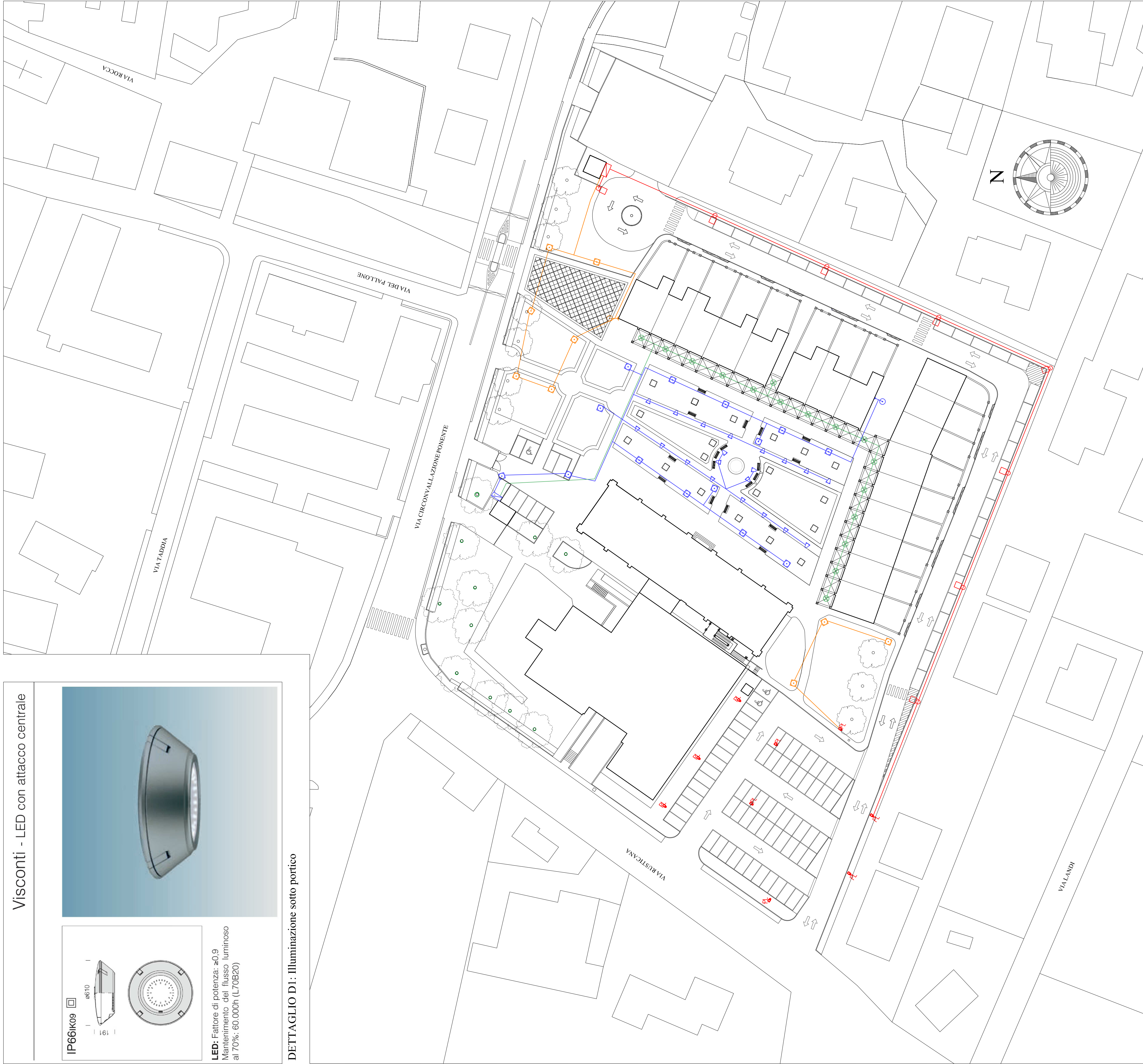
PLANIMETRIA DI PROGETTO, Scala 1:500
